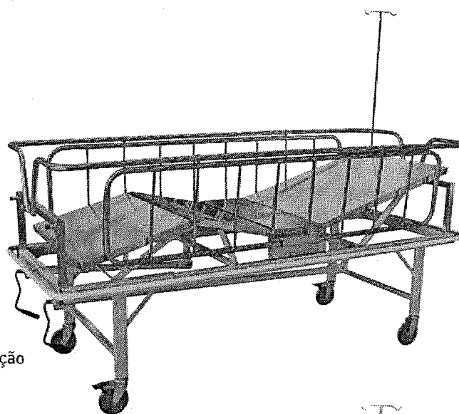
MD 050B | Cama Fowler de Recuperação e UTI ■ com 03 manivelas (Proclive ou Elevação do Leito)
