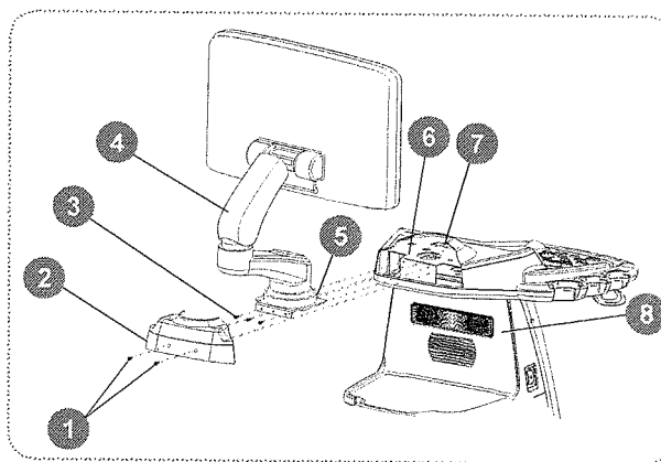
Figura 3-1 Montagem do Sistema
