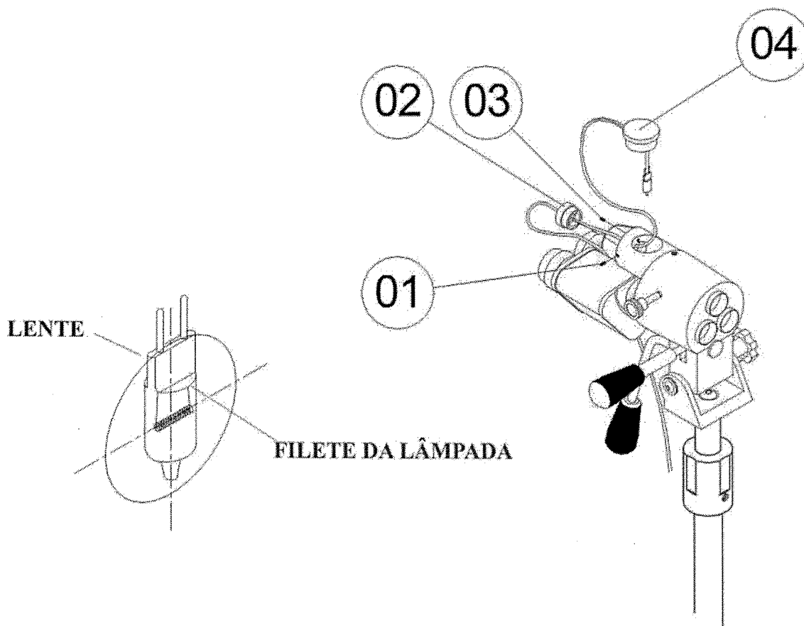
Figura 7 – Substituição da lâmpada 20W
