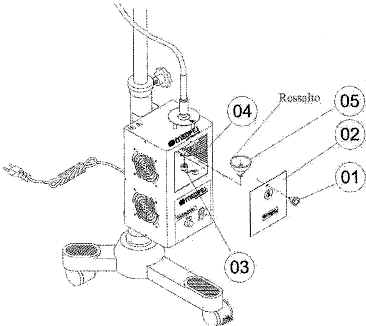
Figura 8 – Substituição da lâmpada 150W
