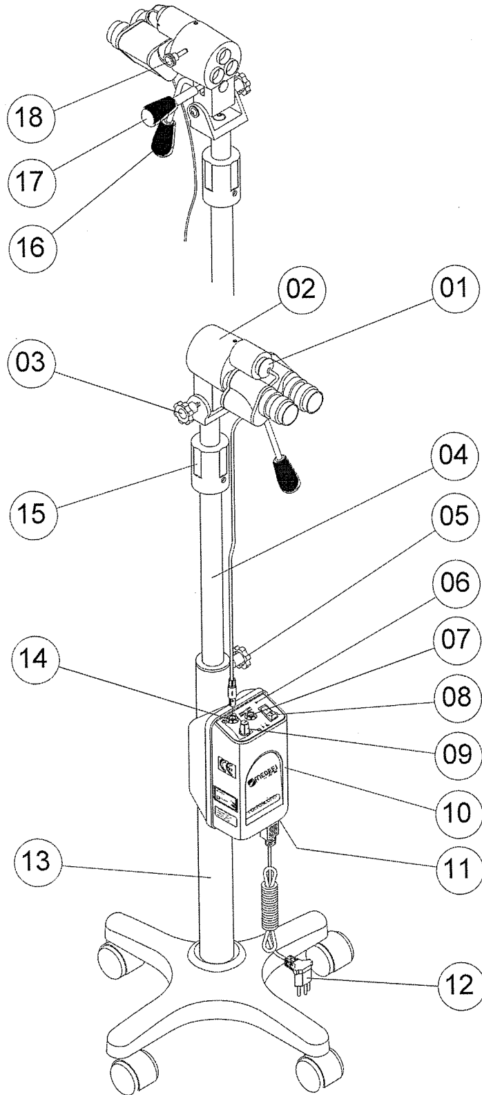
Figura 2 - Colposcópio binocular PE-7000 F
