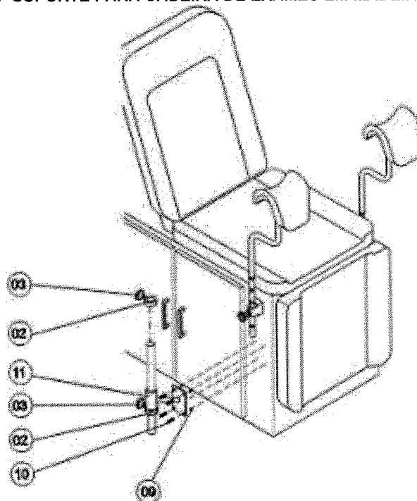
Figura 1 – Montagem dos acessórios PE-7000 F / PE-7000 V / PE-7000 Z
